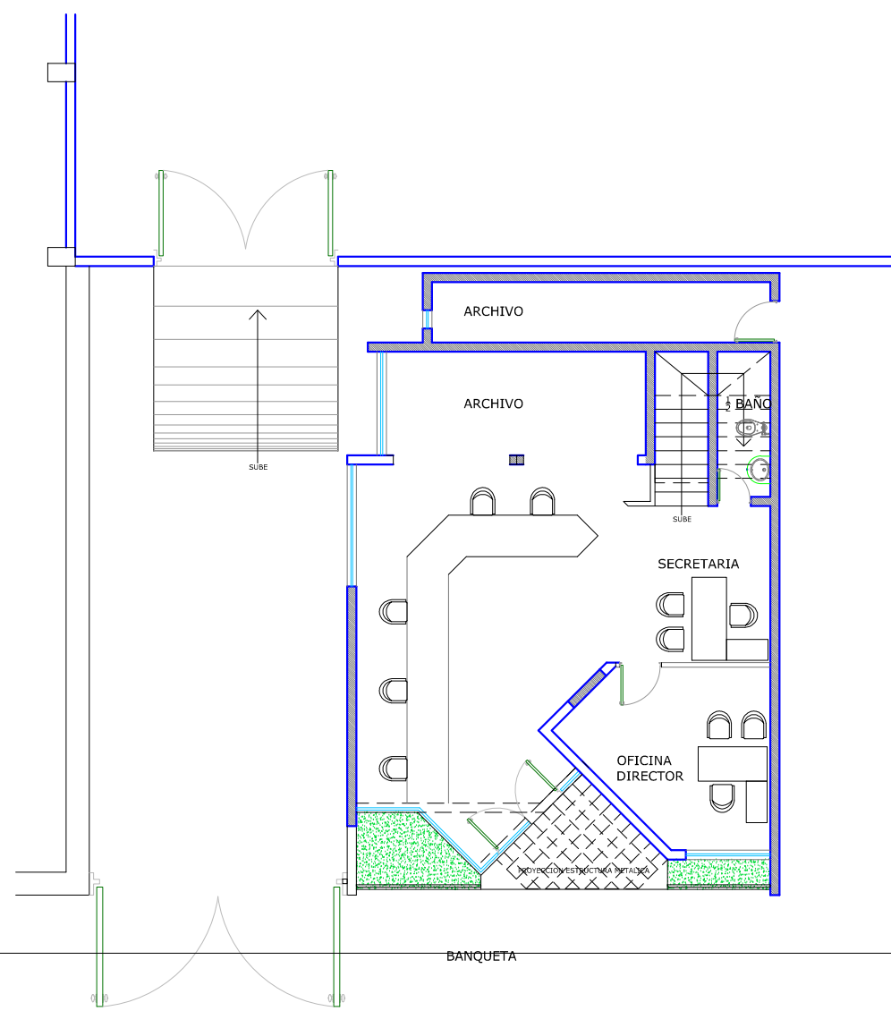
PLANTA BAJA ARQUITECTONICA PROPUESTA.
