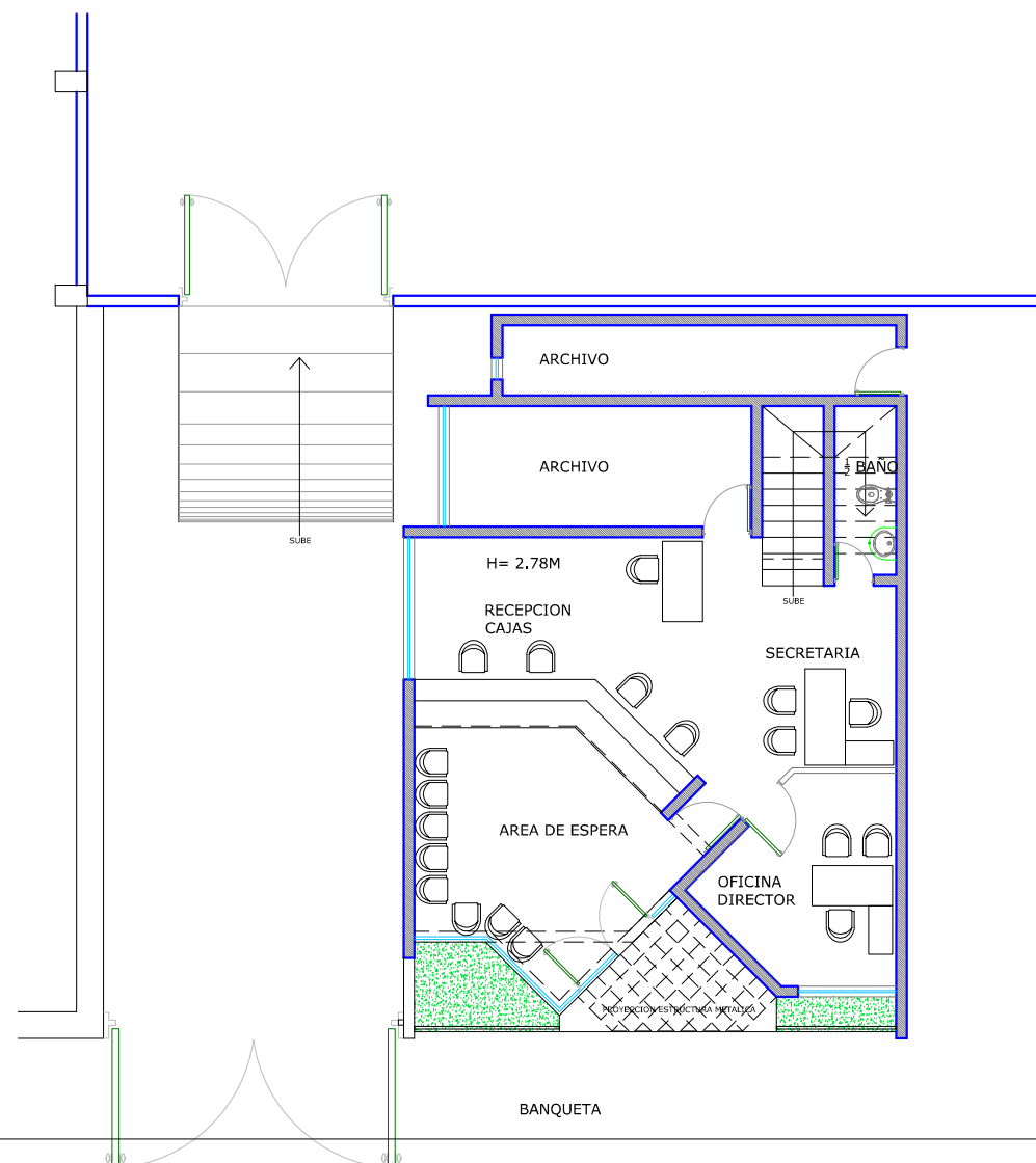
PLANTA BAJA ARQUITECTONICA ESTADO ACTUAL
